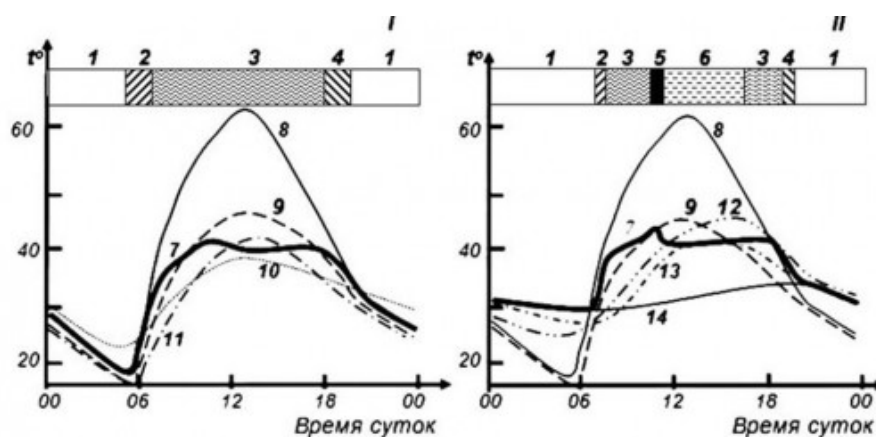
Рис. 5. Динамика температур среды и тела ящериц в Каракумах в летний период: 1 – полосатая ящурка; II – песчаная круглоголовка. Общие формы поведения ящериц: 1 – ночной отдых, 2 – нагревание, 3 – the thermal ТСП, 4 – остывание, 5 – добровольный перегрев, 6 – дневной отдых. Температуры: 7 – тела ящериц; 8 – поверхности почвы на открытом месте; 9 – воздуха в приземном слое (на высоте 2 см) на открытом месте; 10 – воздуха в кроне дерева на высоте 2 м; 11 – поверхности почвы в тени кустов; 12 – почвы на глубине 5 см; 13 – почвы на глубине 10 см; 14 – почвы на глубине 15 см
