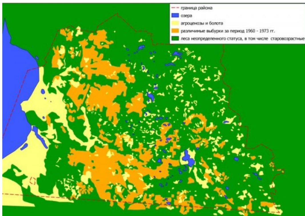
Рис. 2. Территории вырубok в 1960-1973 гг.
