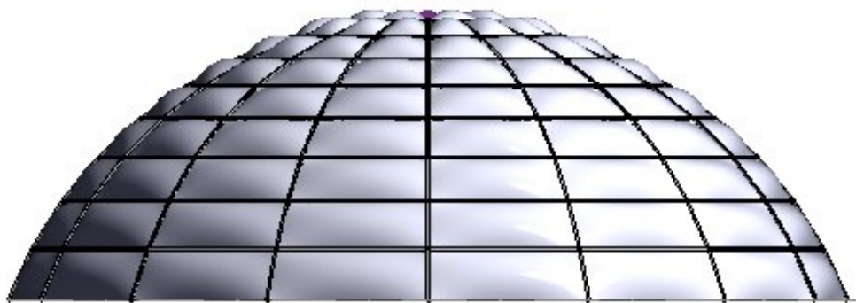
Рис.4 Архитектурная модель
