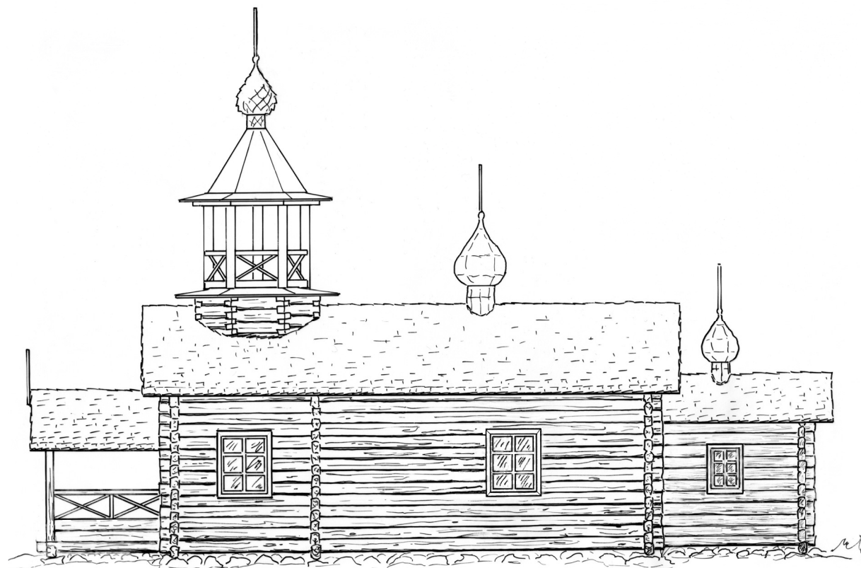
Рис. 7. Реконструкция церкви/часовни Св. Петра в Гафострове. Южный фасад. Рис. А. Яскеляйнена, И. Переходовой
