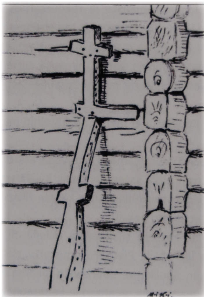
Рис. 5. Фрагмент стены. Рубка в охряпку с полной отёской. Рис. Мери Кюрки, 1941 г.
