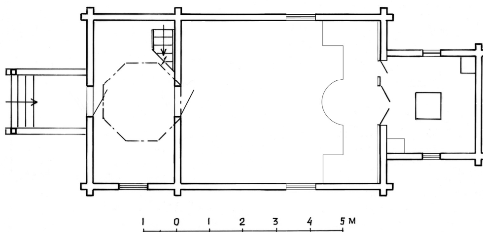
Рис. 6. Реконструкция церкви/часовни Св. Петра в Гафострове. План
