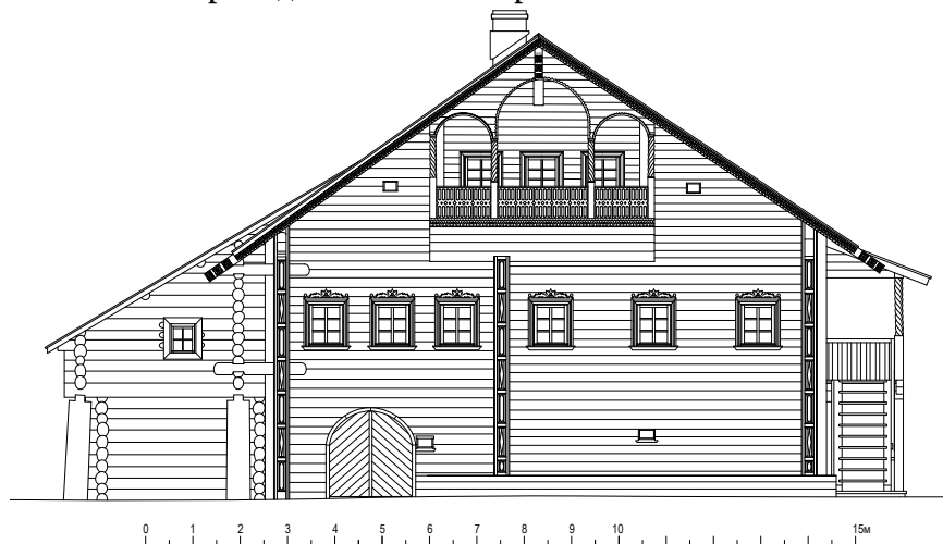
Дом Абрамовых в дер. Сычи. Графическая реконструкция западного, лицевого, фасада
